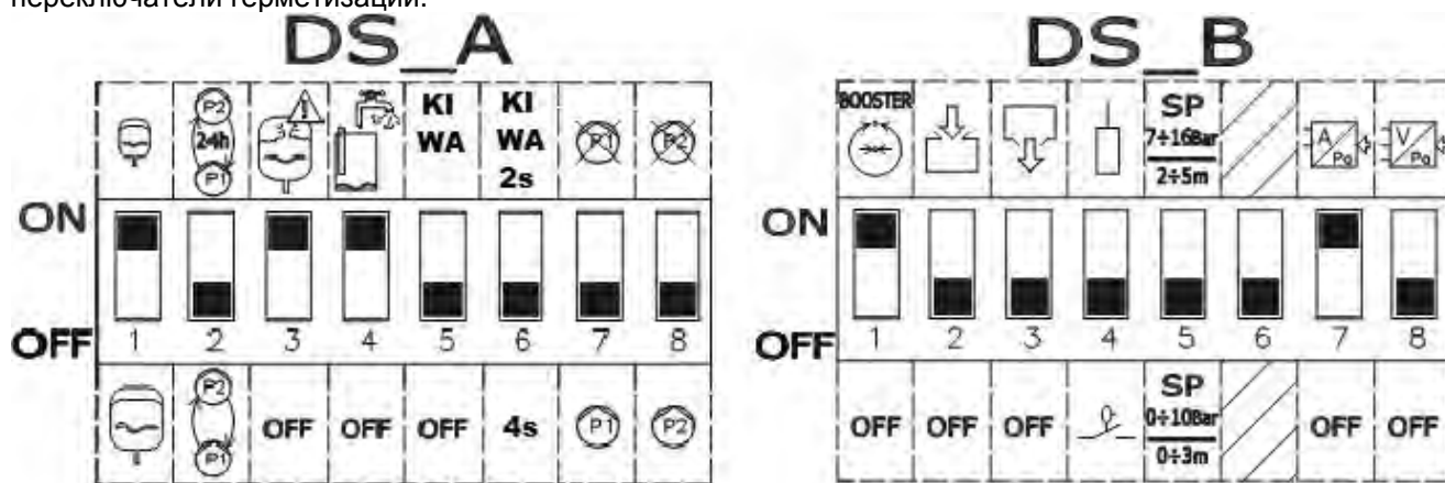
Схема 14: Dip-переключатели герметизации
