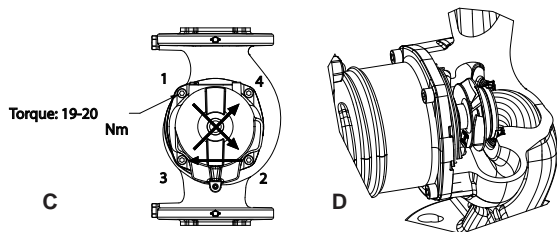
Сх 2: Инструкции по монтажу головок двигателя
