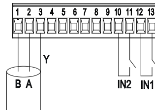
Сх. 7: Съемная клеммная колодка 13 полюсов: цифровые вводы и MODBUS
