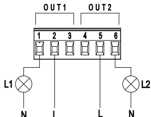
Сх. 9: Съемная клеммная колодка 6 полюсов: пример подсоединения выводов
